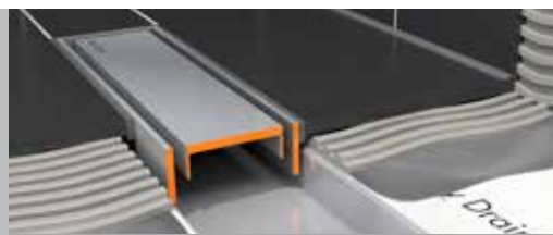
Espesor de la baldosa 7 - 18 mm
